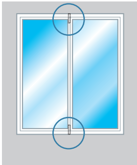
VERROUS HAUT ET BAS DE MAINTIEN DU VANTAIL SECONDAIRE POUR LES PORTES-FENÊTRES
